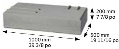
MODULE DE COIN
