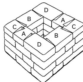
STEP 4 : rows 4 and 8
