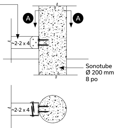
COUPE A-A
