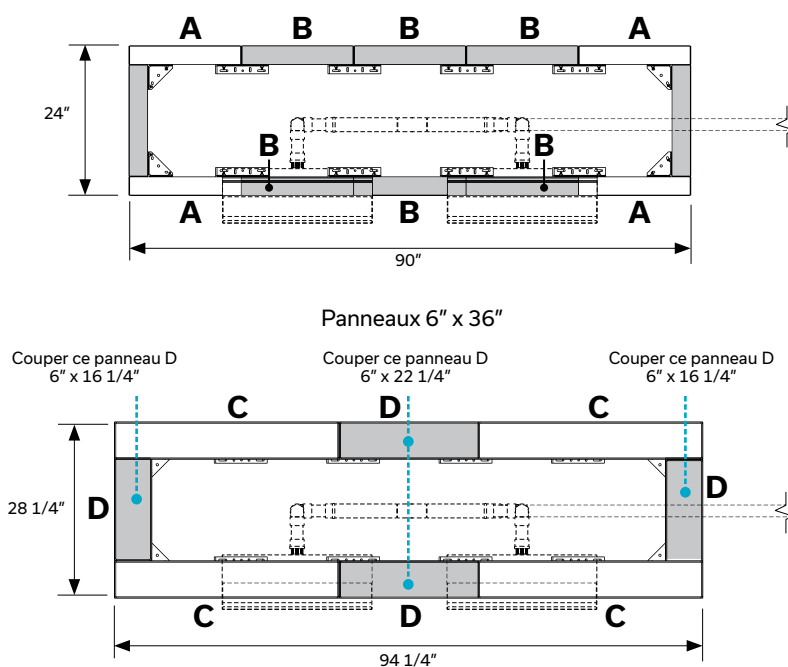
VUE DU HAUT Panneaux 18" x 36"
