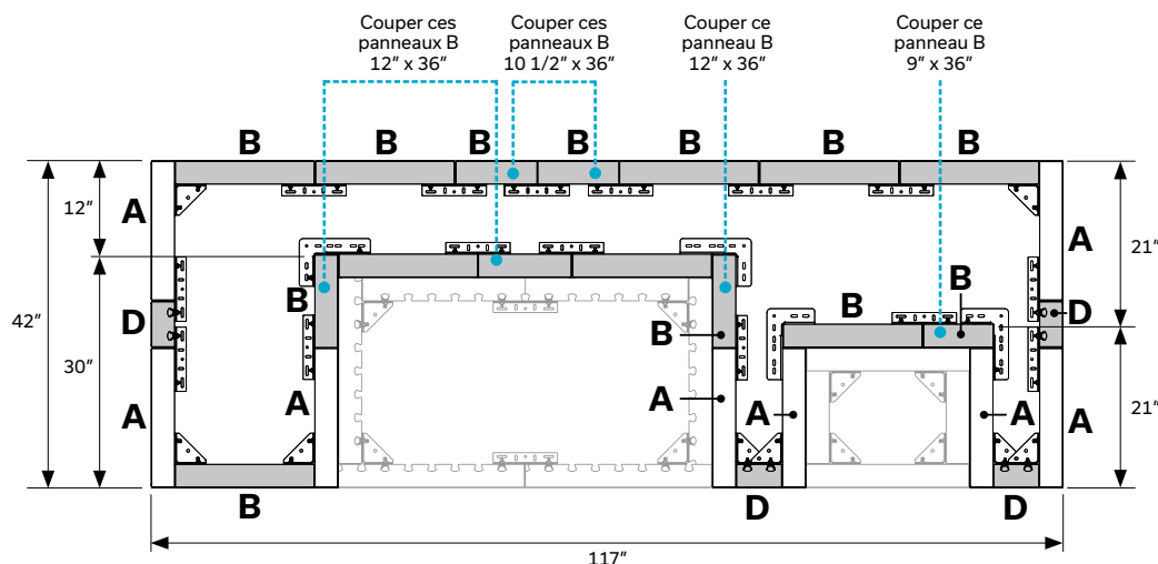
VUE DU HAUT
