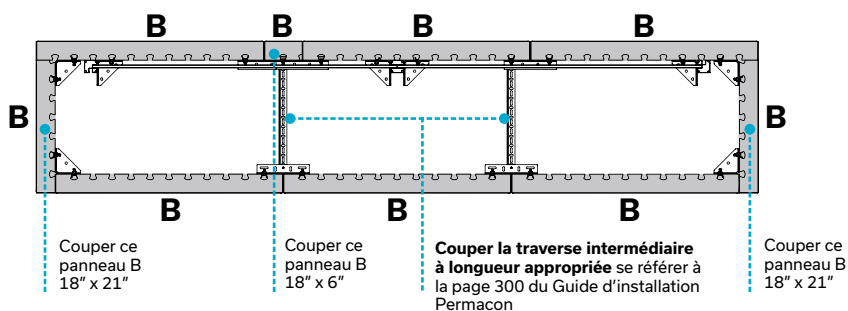
Panneaux 6 x 36 po
