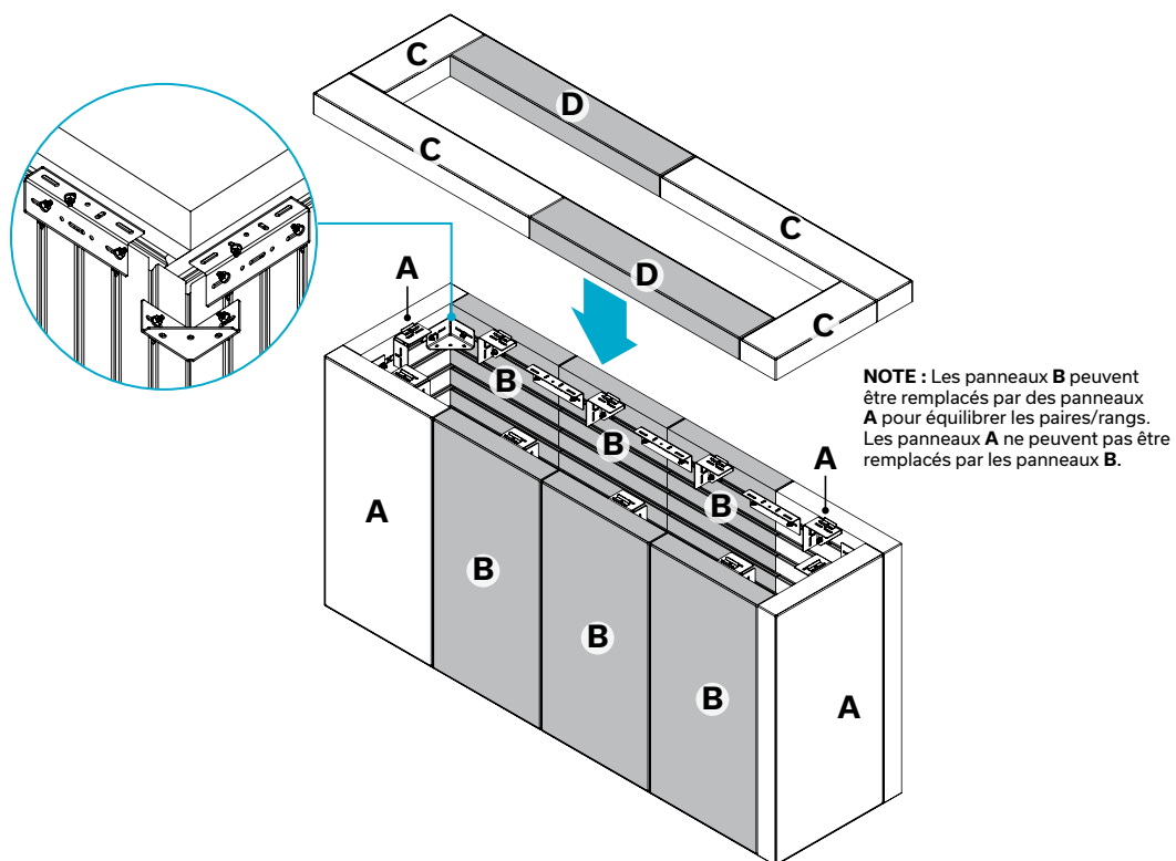
VUE DU HAUT Panneaux 18 x 36 po
