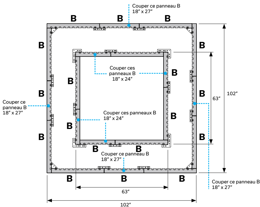
VUE DU HAUT
