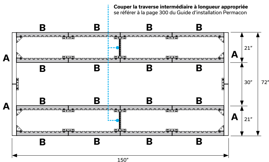
VUE DU HAUT
