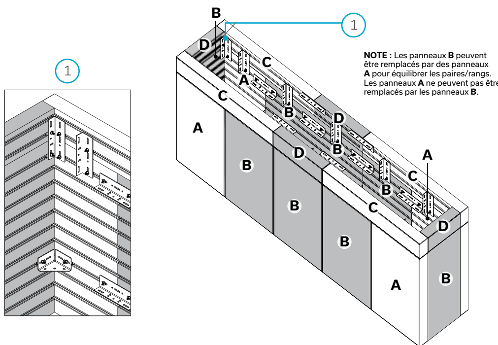
VUE DU HAUT Panneaux 18 x 36 po
