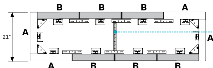
Panneaux 6 x 36 po
