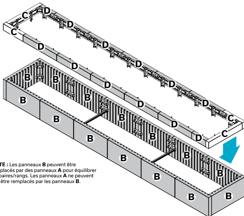
VUE DU HAUT Panneaux 6 x 36 po
