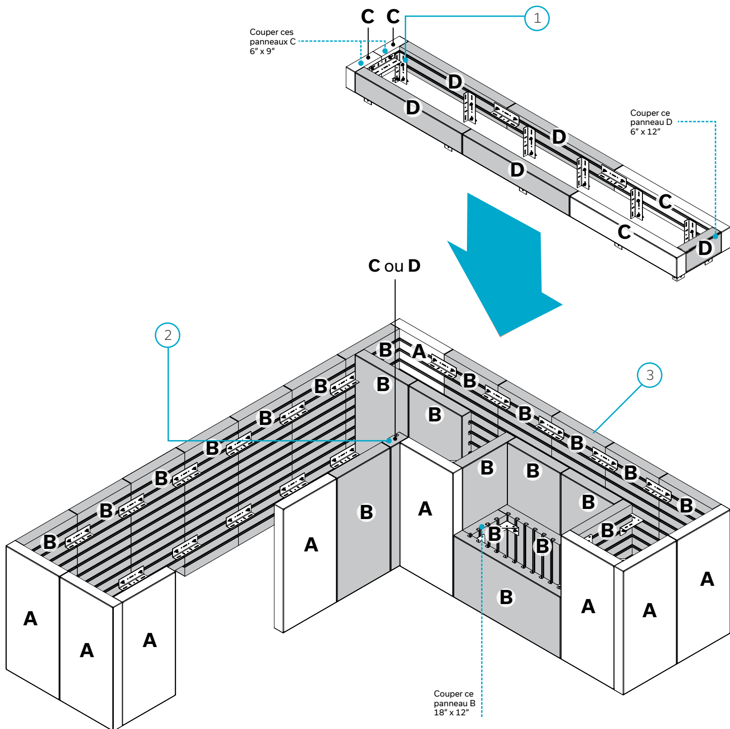
VUE ÉCLATÉE
