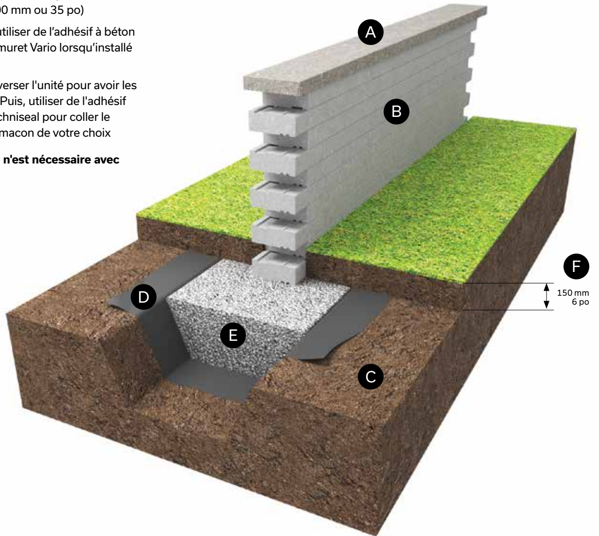
VUE ISOMÉTRIQUE
