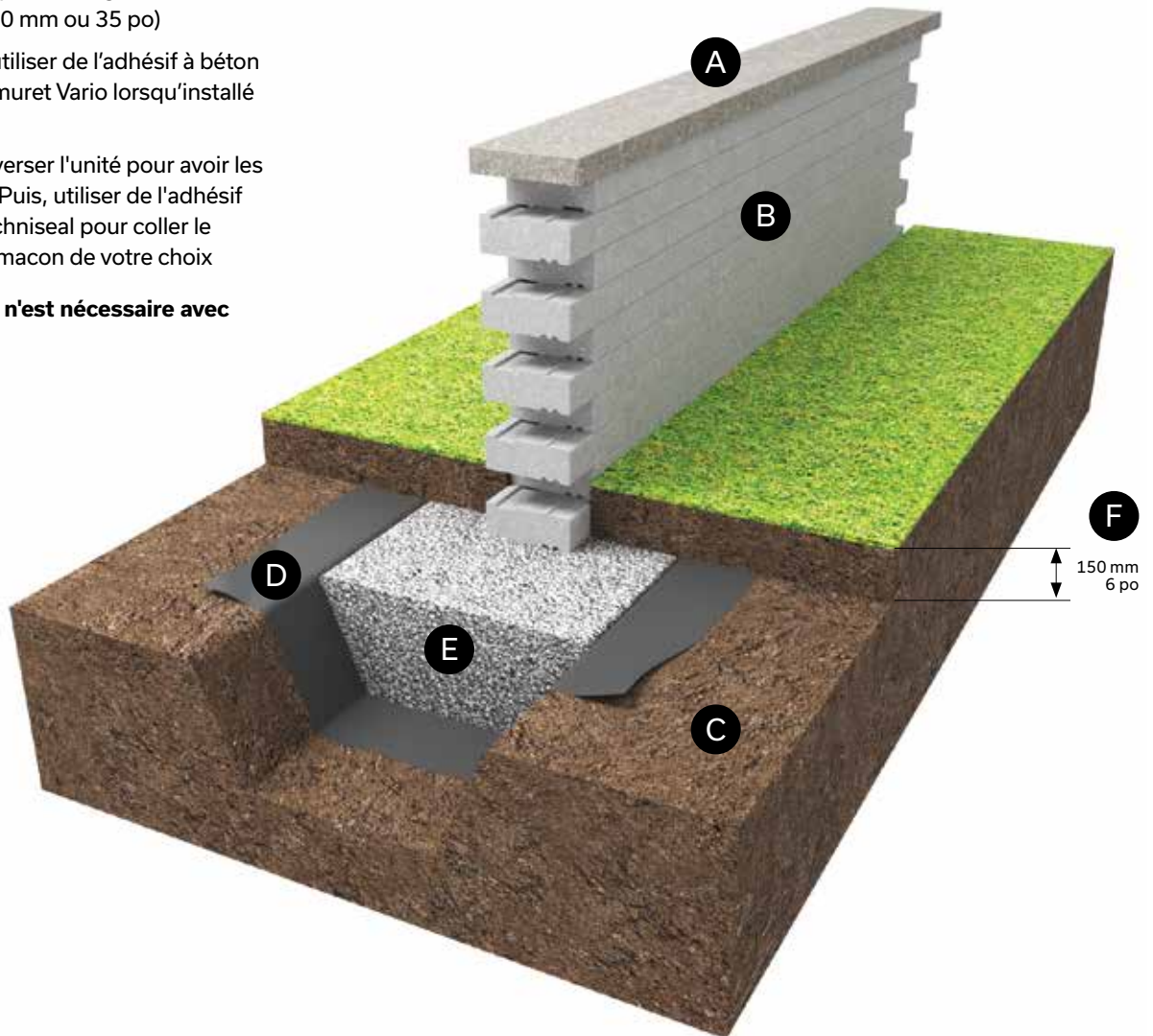
VUE ISOMÉTRIQUE
