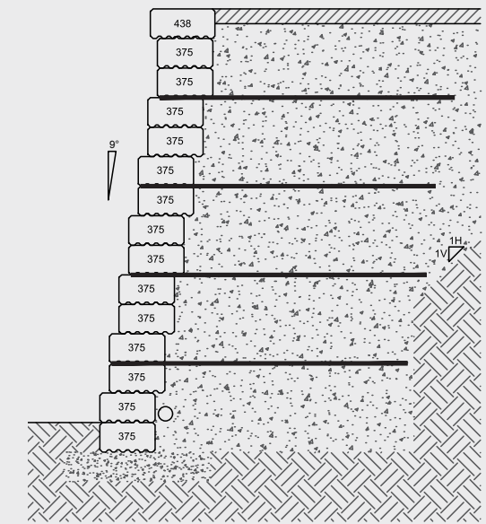
Muret Grande Lisse 3 m (9,8 pi) 15 rangs incliné 9° renforcé
