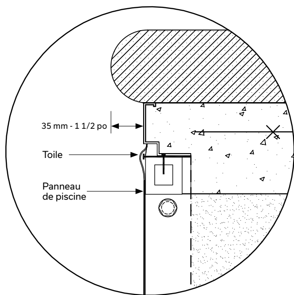
DÉTAIL 1
