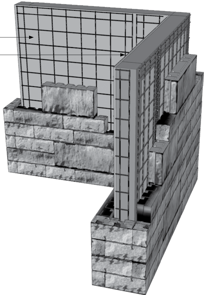
EXEMPLE DE CONTREVENTEMENT (écran camouflage)
