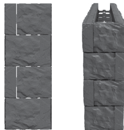
VUE EN ÉLEVATION
