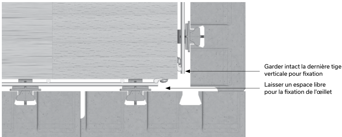
COUPE DE LA GRILLE (VUE EN PLAN)
