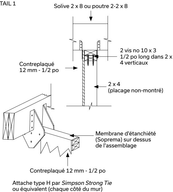
DÉTAIL 1
