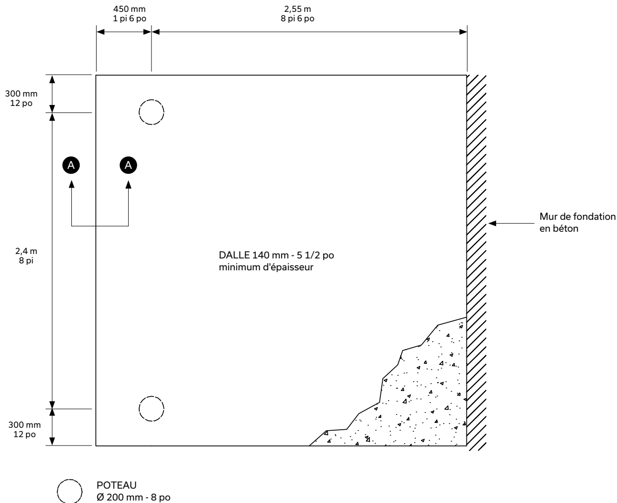
Juque de patio de béton VUE EN PLAN
