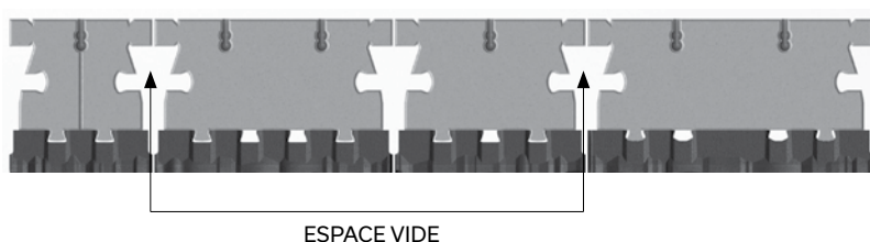
Muret lafitt tandem (VUE EN PLAN)
