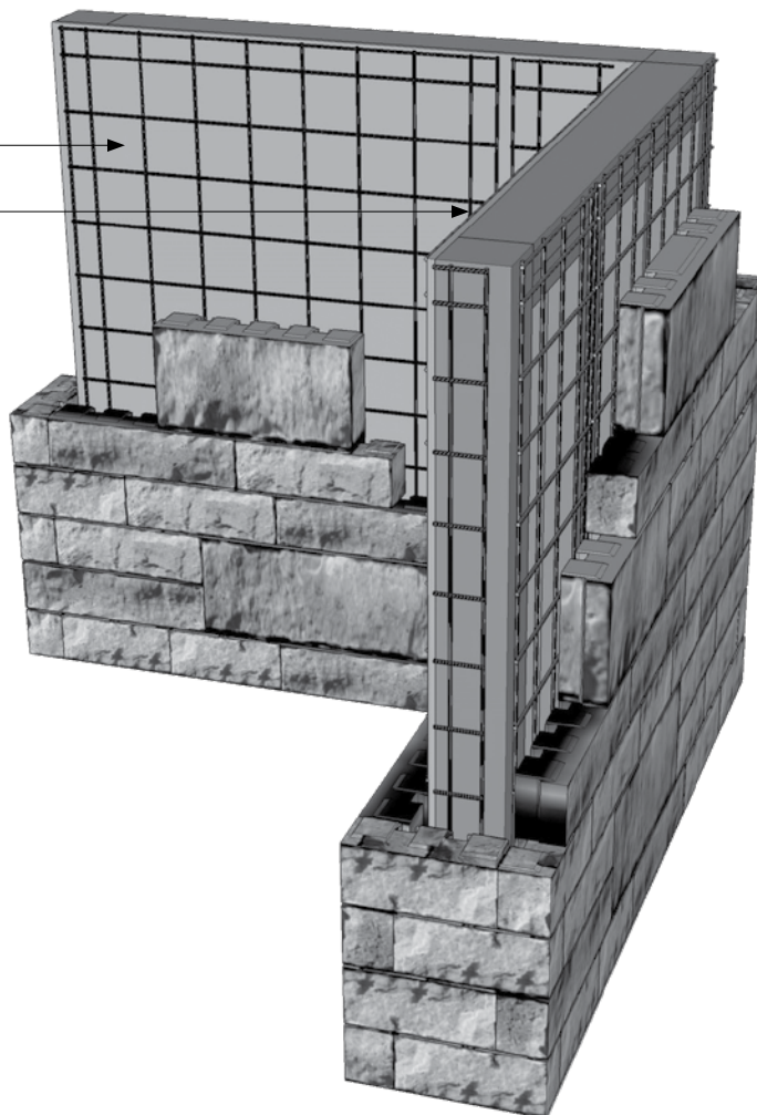
EXEMPLE DE CONTREVENTEMENT (écran camouflage)
