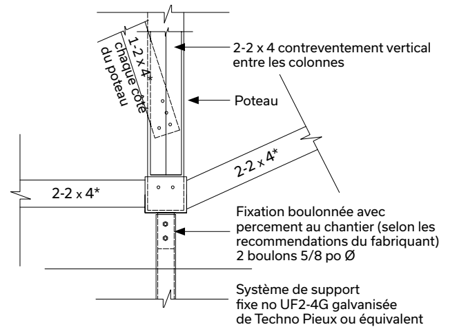
DÉTAIL 2
