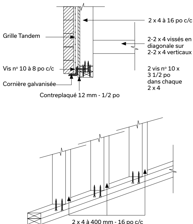
DÉTAIL 3
