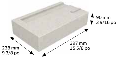
MODULE DE COIN MOYEN - GAUCHE
